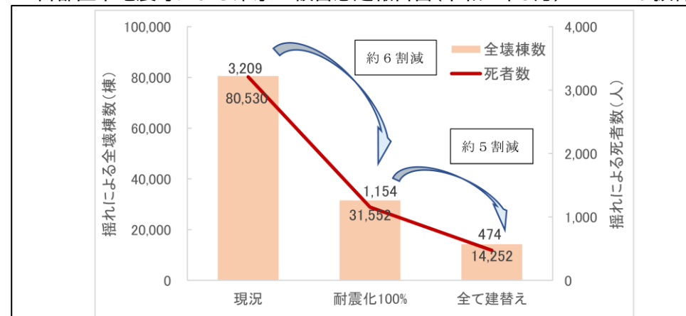
図 耐震化による対策効果(都心南部直下地震)
