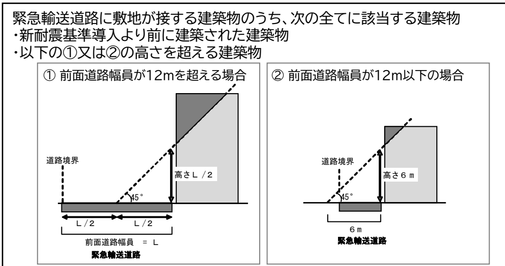
図10 沿道建築物の要件
