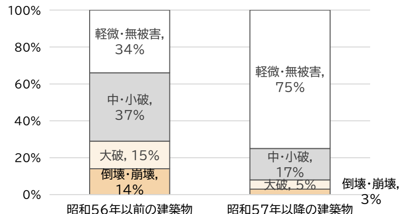
図4 阪神・淡路大震災における昭和56年以前と昭和57年以降に建築された建築物の被害状況
