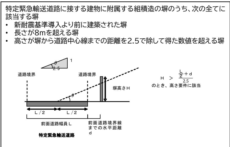
図11 特定緊急輸送道路沿いの塀の要件
