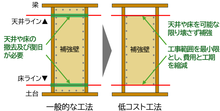
図34 低コスト工法のイメージ
