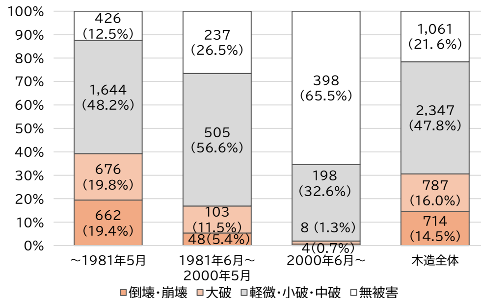
図5 木造建築物の建築時期別の被害状況
