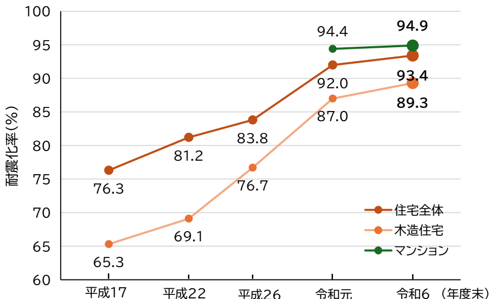
図32 耐震化率の推移(新耐震基準)
