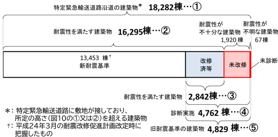
図19 特定緊急輸送道路沿道の建築物の耐震化状況(令和7年12月末時点)
